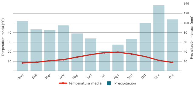
Climograma de Oviedo
